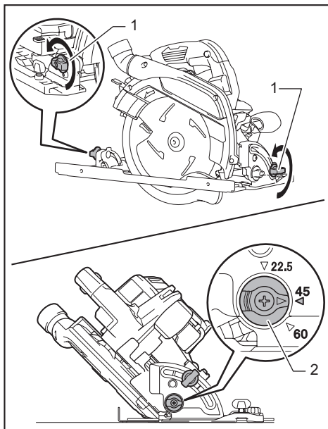
► 1. Vis de serrage 2. Butée fixe
