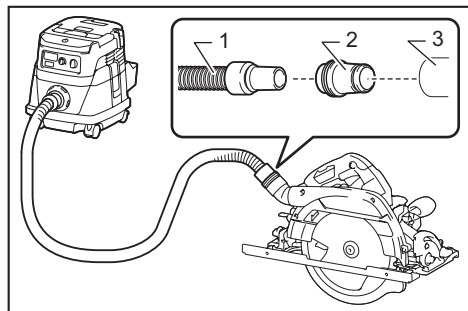
► 1. Manguera de la aspiradora 2. Manguitos delanteros 24 3. Boquilla para polvo
