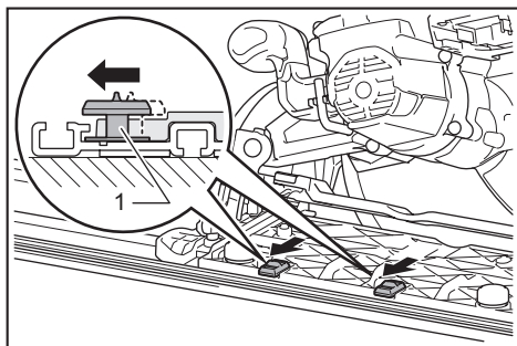
► 1. Palanca deslizante
