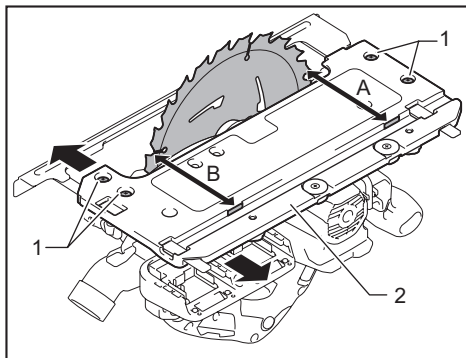
► 1. Screw 2. Base
